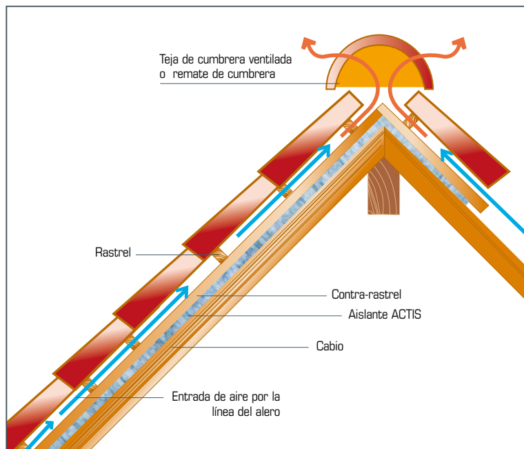
Ventilación mediante entrada de aire por la línea del alero y salida superior en la cumbre
