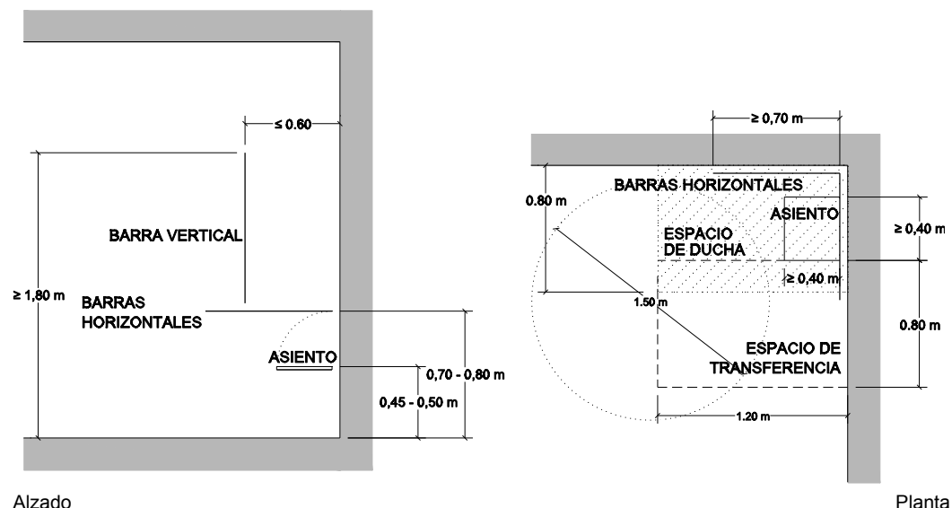
Alzado
