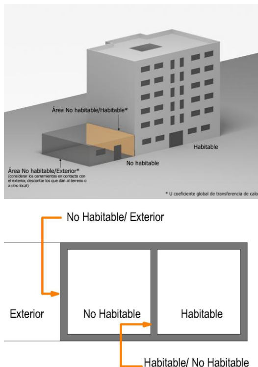
Imagen 26 Esquema áreas de muro en contacto con espacios no habitables
