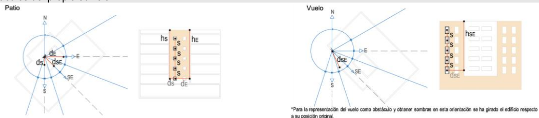
Imagen 21 Sombras por obstáculos remotos o del propio edificio. Sureste
