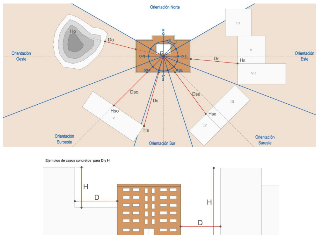
Imagen 5 Características de los obstáculos del entorno
