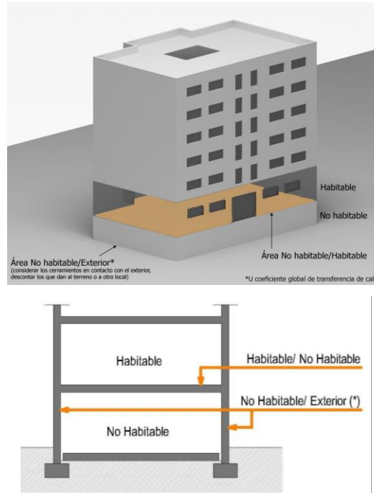
Imagen 39 Esquema áreas de suelo en contacto con espacios no habitables
