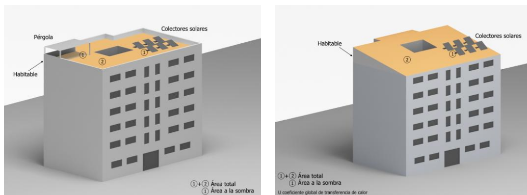
Imagen 29 Esquema áreas de cubierta en contacto con ambiente exterior- Plana e inclinada
