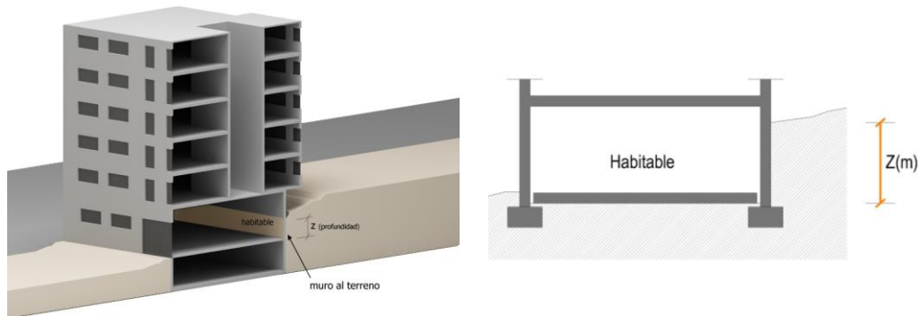
Imagen 25 Esquema áreas de muro en contacto con el terreno
