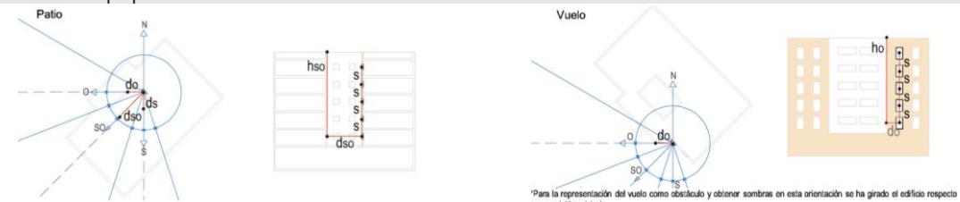
Imagen 18 Sombras por obstáculos remotos o del propio edificio. Suroeste
