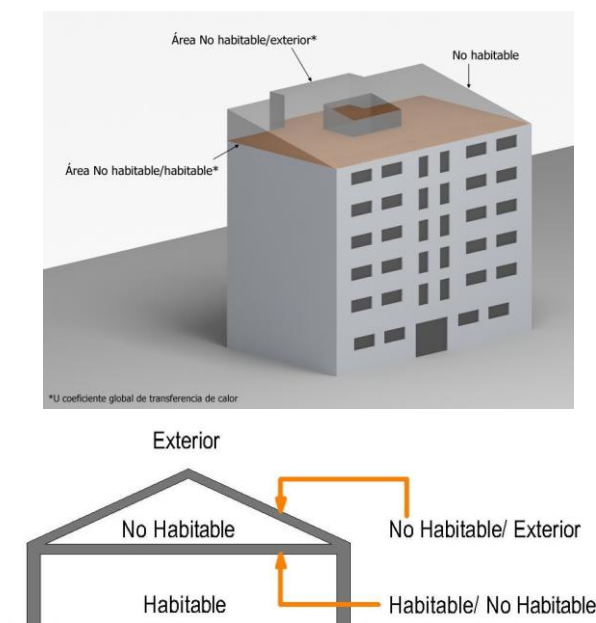
Imagen 30 Esquema áreas de cubierta en contacto con espacio no habitable
