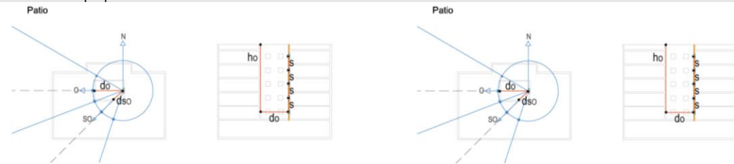
Imagen 17 Sombras por obstáculos remotos o del propio edificio. Oeste
