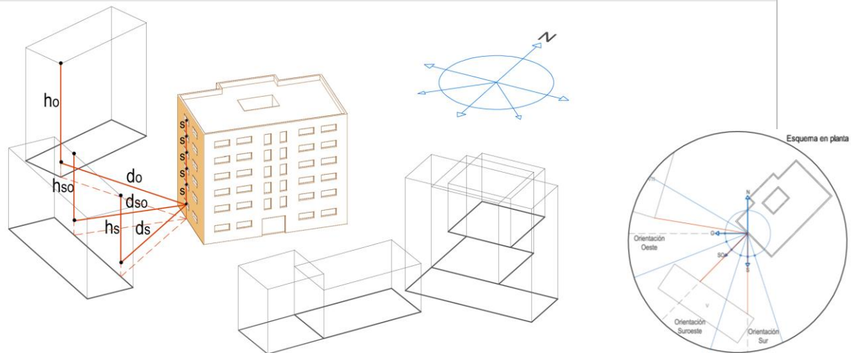
Imagen 17 Sombras por obstáculos remotos o del propio edificio. Oeste
