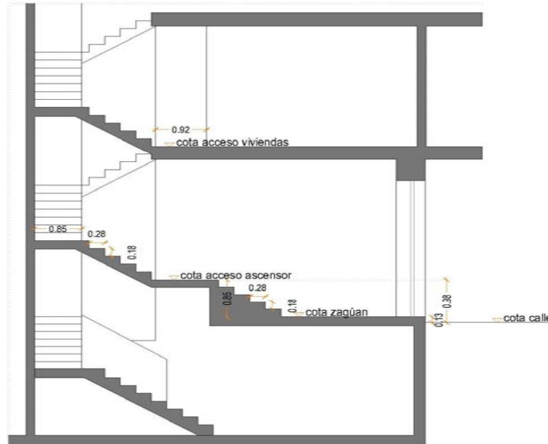
Sección tipo, zaguán y acceso viviendas
