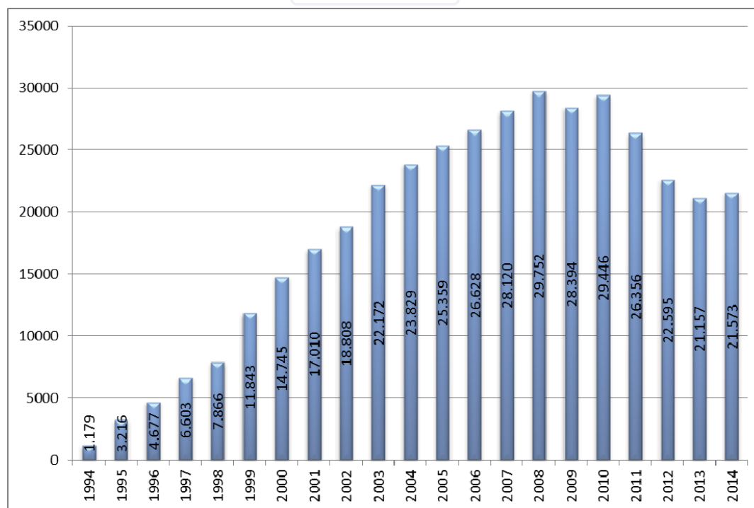
Gráfico 5: Recogida separada papel/cartón (t)
