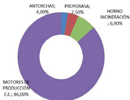
Gráfico 4: Destinos del biogás captado
