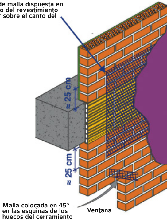
-Detalle 8- Encuentros de la hoja exterior con el canto de forjado y con los huecos de fachada
