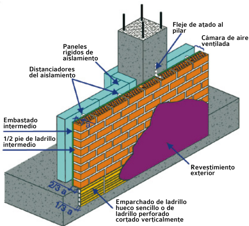
-Detalle 1- Apoyo y anclaje de la hoja exterior de una fachada con fábrica de \frac{1}{2} pie de ladrillo perforado
