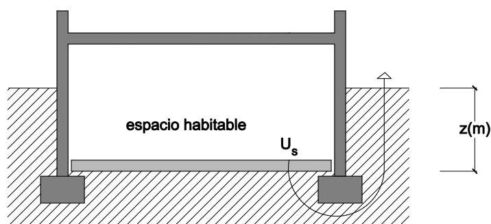
Figura 2 Solera enterrada
