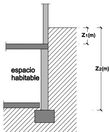
Figura 4 Muro enterrado
