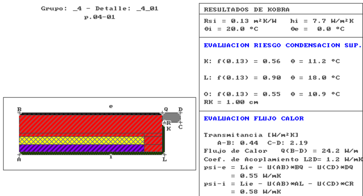
Figura 1. Evaluación de los flujos de calor con el programa Kobra
